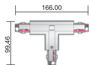
“T”接頭左2 Pro-0436 左二 三向接駁器“左二”
