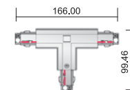
Pro-0436 右二 “T”接頭“右二” 三向接駁器“右二”
