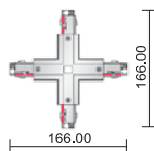
Pro-0437 “+”接頭 四向接駁器
