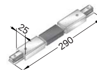
Pro-0239 軟接頭 2線角度接駁器使用
